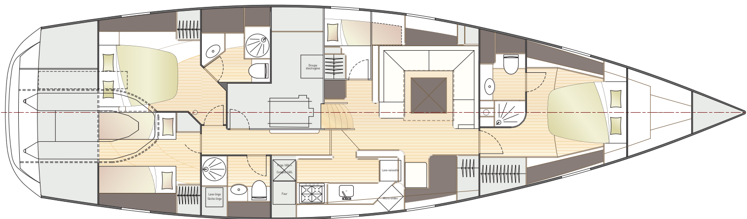
Aménagement intérieur 4 cabines / Inside layout with 4 cabins
