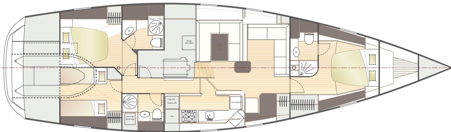
Aménagement intérieur 3 cabines / Inside layout with 3 cabins
