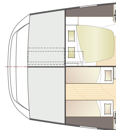
Aménagement sans garage à annexe Layout without tender garage
